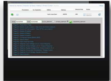
Reportes selectivos
